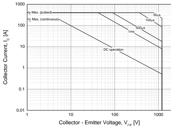
Fig. 11 SOA
